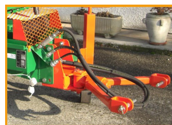
Attelage bras de relevage
